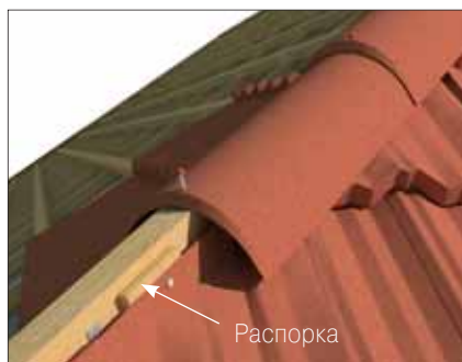
Вариант 2: Вальмовый брус с распоркой
