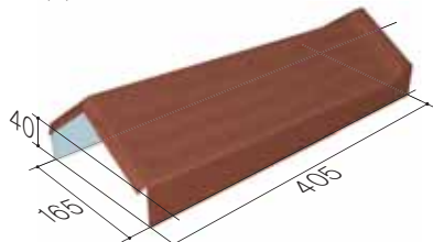
ТРЕУГОЛЬНЫЙ КОНЕК Эффективная длина: 370 мм
