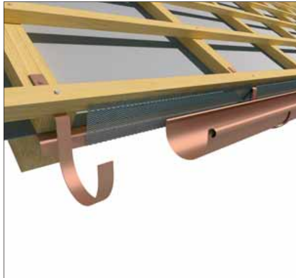
Вариант 1: Карнизная планка уходит за водосток
