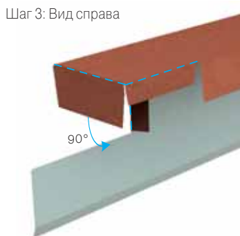
Шаг 3: Вид справа
