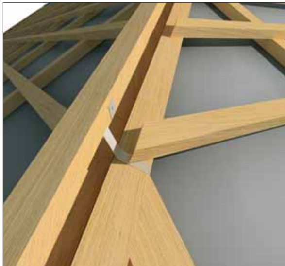
Вариант 1: Коньковый брус - монтаж с коньковыми кронштейнами
