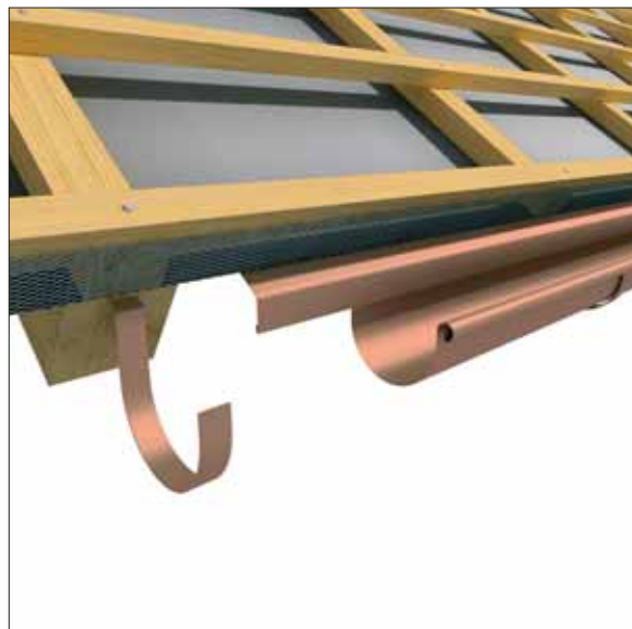
Вариант 2: Карнизная планка заходит в водосток
